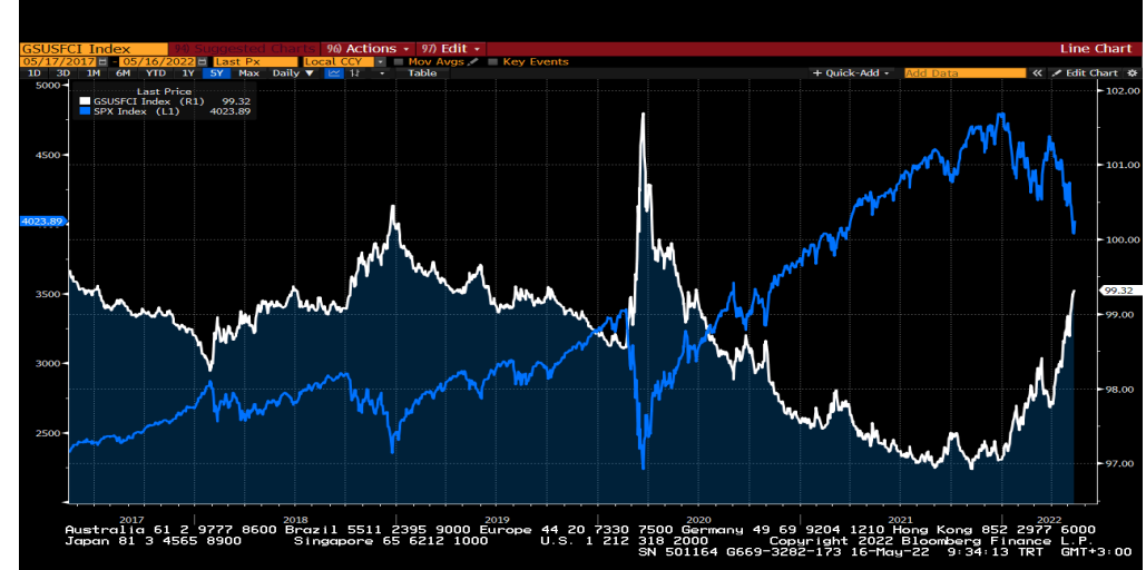
ABD finansal koşullar endeksi (beyaz seri) ve S&amp;P500 son 5 yıllık seyri...
