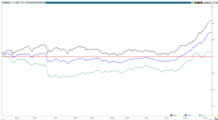
XU100—XUSIN—XBANK 2021 performansları (%)
