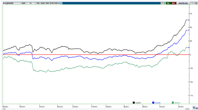
XU100—XUSIN—XBANK 2021 performansları (%)
